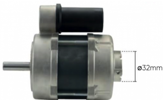
Moteur brûleur 110W 230V-50Hz, avec moyeu diam 32 câble 50 cm
